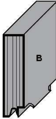
RAINURÉ FEMELLE POUR CHARNIÈRE ENCASTRÉE
