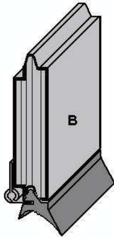
RAINURÉ MÂLE/FEMELLE POUR CHARNIÈRE ENCASTRÉE
